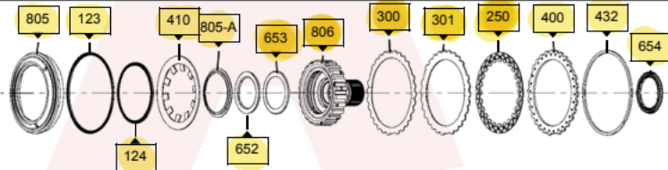
'A' Clutch
