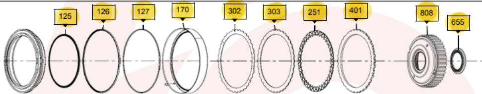
'B' Clutch
